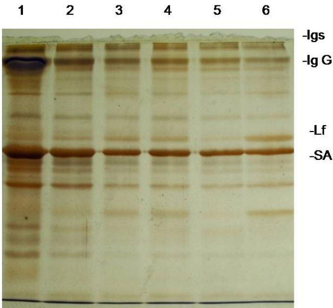
Figura 1: SDS-PAGE de lactoserum de Tapirus terrestris a partir del nacimiento de la cría hasta el día 36 posparto. 1: día cero (nacimiento); 2: día tres de lactación; 3: día siete de lactación; 4: día 11 de lactación; 5: día 29 de lactación; 6: día 36 de lactación. Se marcan las proteínas identificadas: Inmunoglobulinas (Igs); Inmunoglobulina G (IgG), Lactoferrina (Lf), seroalbumina (SA).
